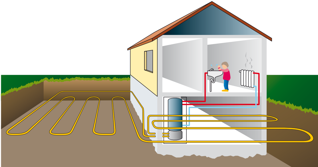
Här ser du ett hus i genomskäring. Huset värms upp med en jordvärmepump som även producerar varmvatten. Värmen hämtas från slingan som ligger nergrävd i jorden. Bild: Bo Reimerdahl
